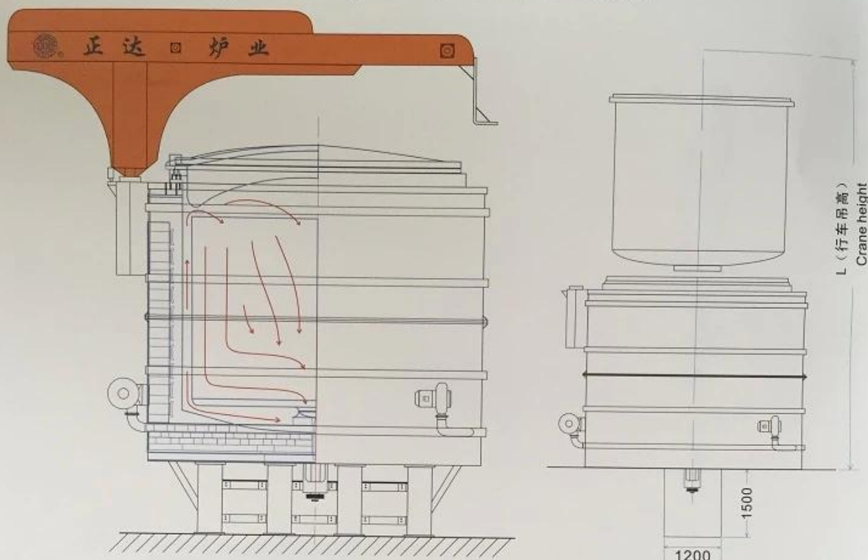
炉体安装吊高（无脚架） Installation lifting of furnace body
